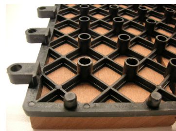
Sous-face en polypropylène avec système d'assemblage par emboîtement
